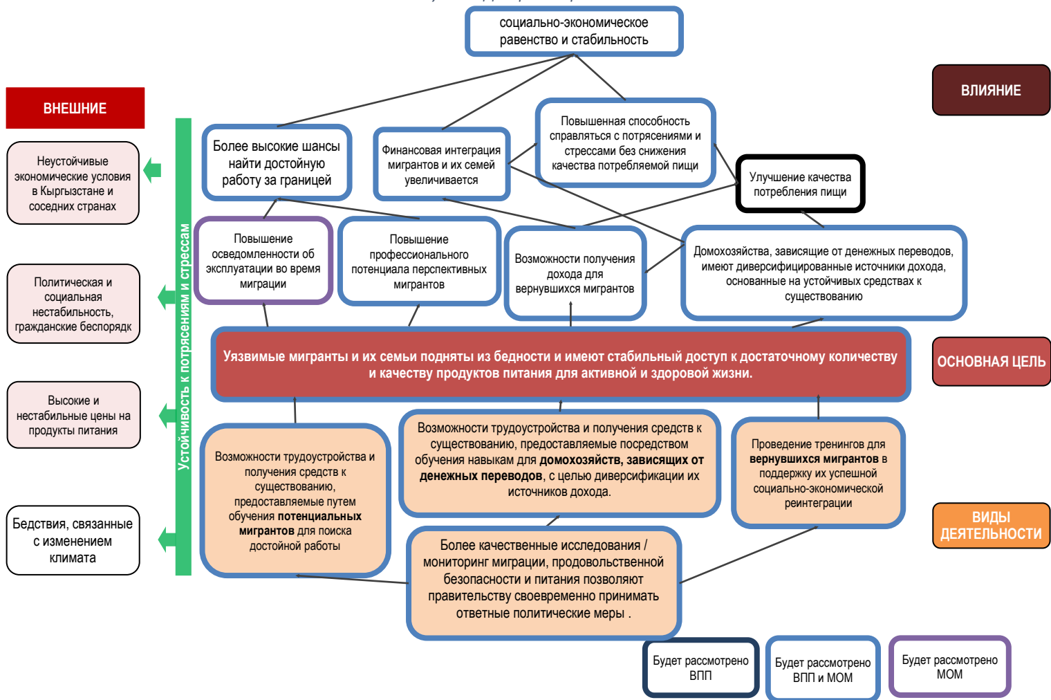
Рисунок 4. Диаграмма решений
